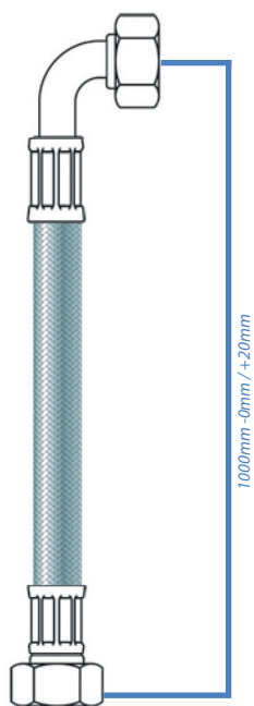
* Vær oppmerksom på at tegning ikke er i realitstiks skala
